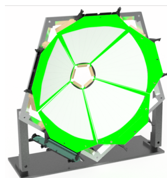
クラスター状態探索のために開発された SAKRA 検出器
